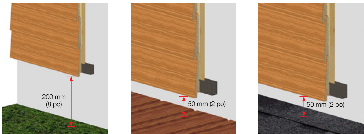
FIGURE 12 • Dégagement minimal du revêtement au-dessus d'une surface
