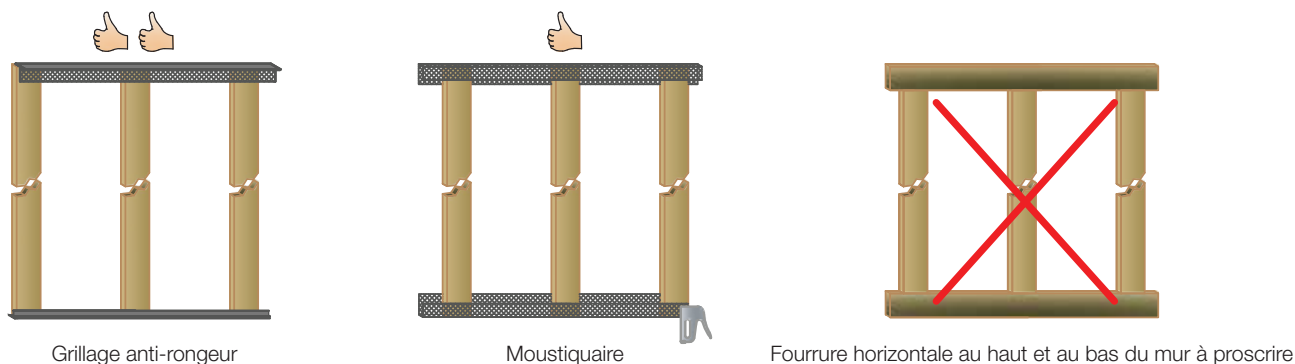
FIGURE 7 • Barrières de protection au bas et au haut des murs
