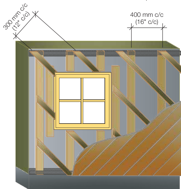
FIGURE 5 • Disposition des fourrures pour le revêtement vertical
