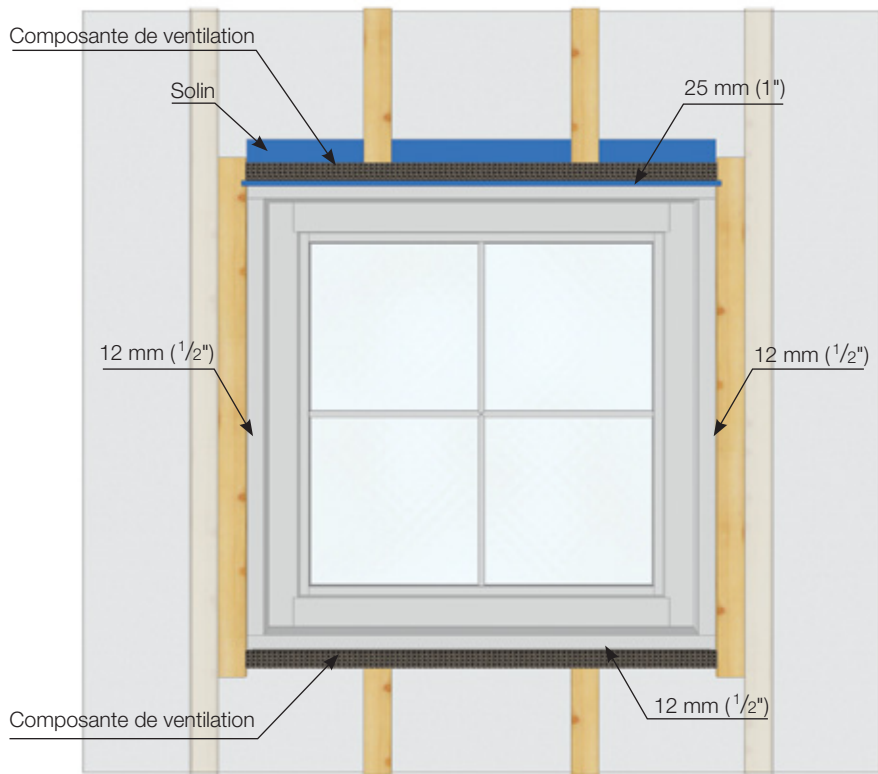
a) Vue de face
