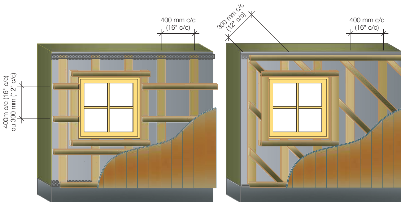
FIGURE 5 • Disposition des fourrures pour le revêtement vertical
