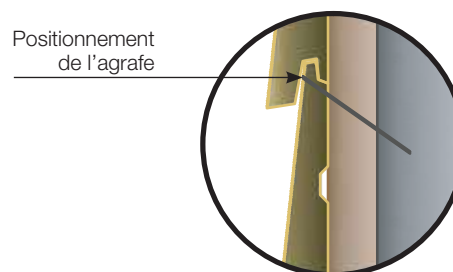
b) Dissimulée par la planche du dessus
