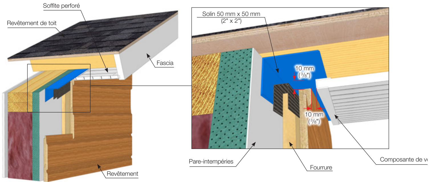
a) En revêtement horizontal
