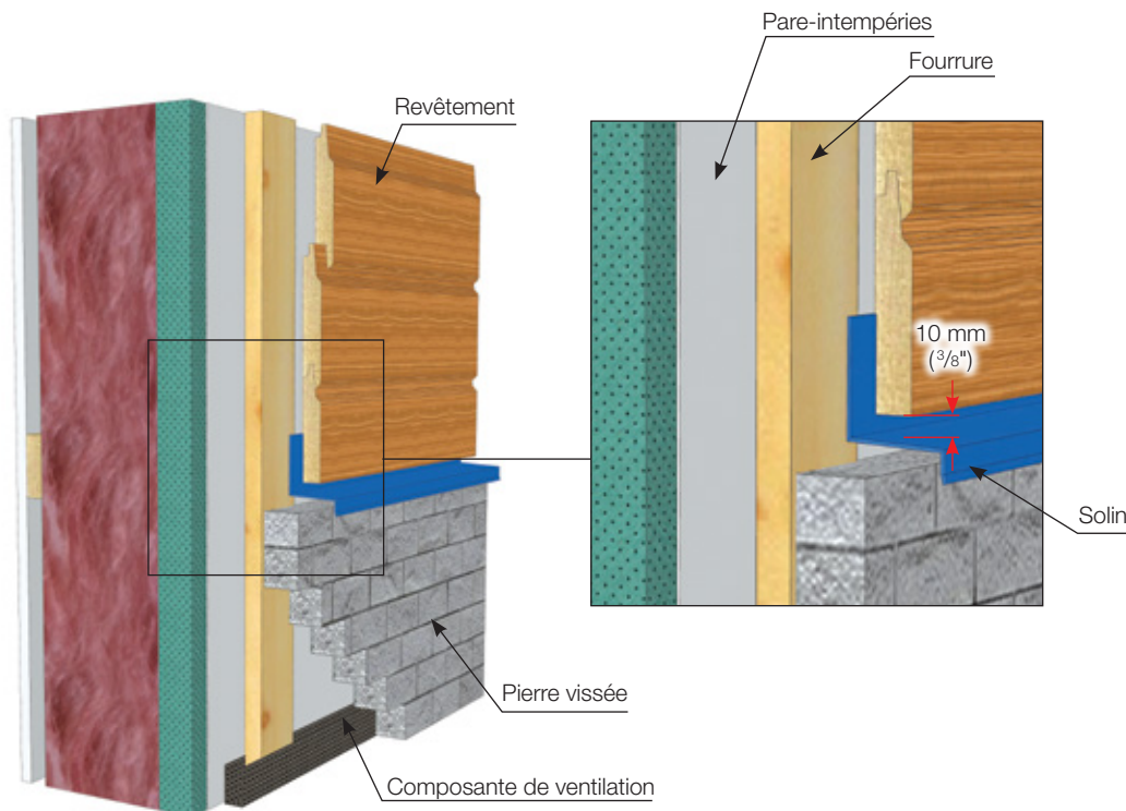
FIGURE 11 • Préparation des murs à la jonction d'un mur de pierres vissées (ou imitation de pierres)
