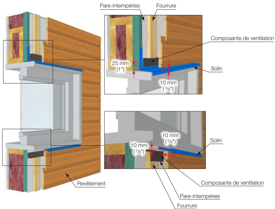
b) Vue en coupe
